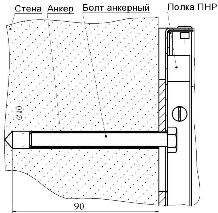
Рисунок 1. Пример крепления полки типа ПНР
