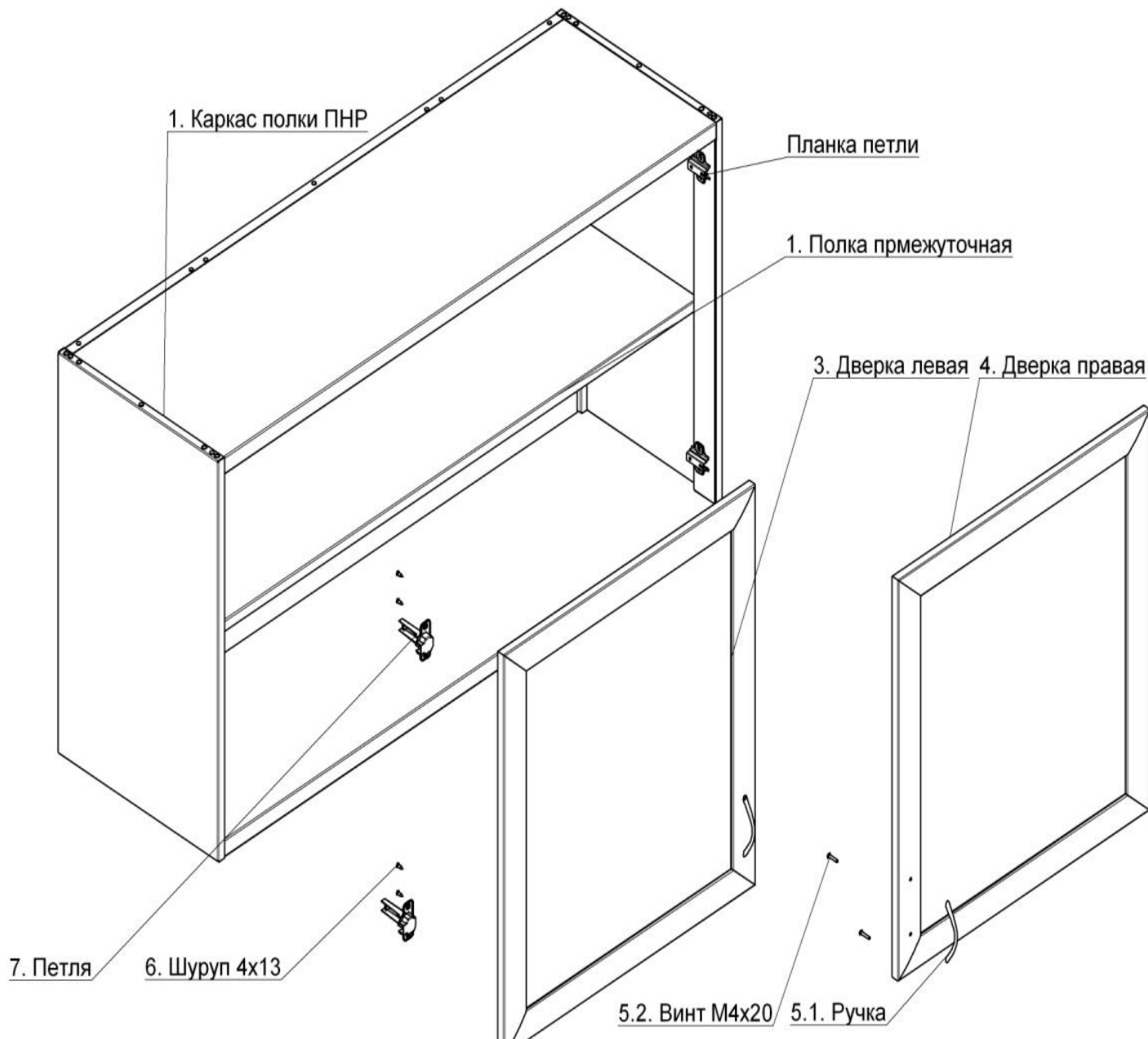
Рисунок 2. Схема для сборки полки типа ПНР.
