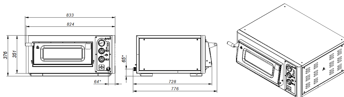
Рис. 3 - Общий вид ПЭП-2
