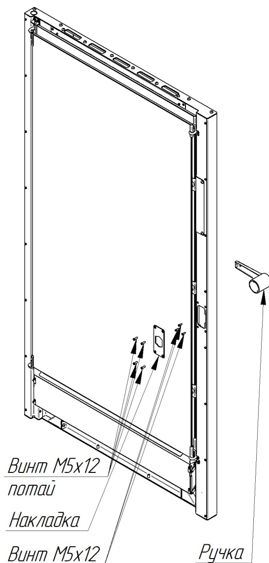
Рис. 11. Замена ручки
