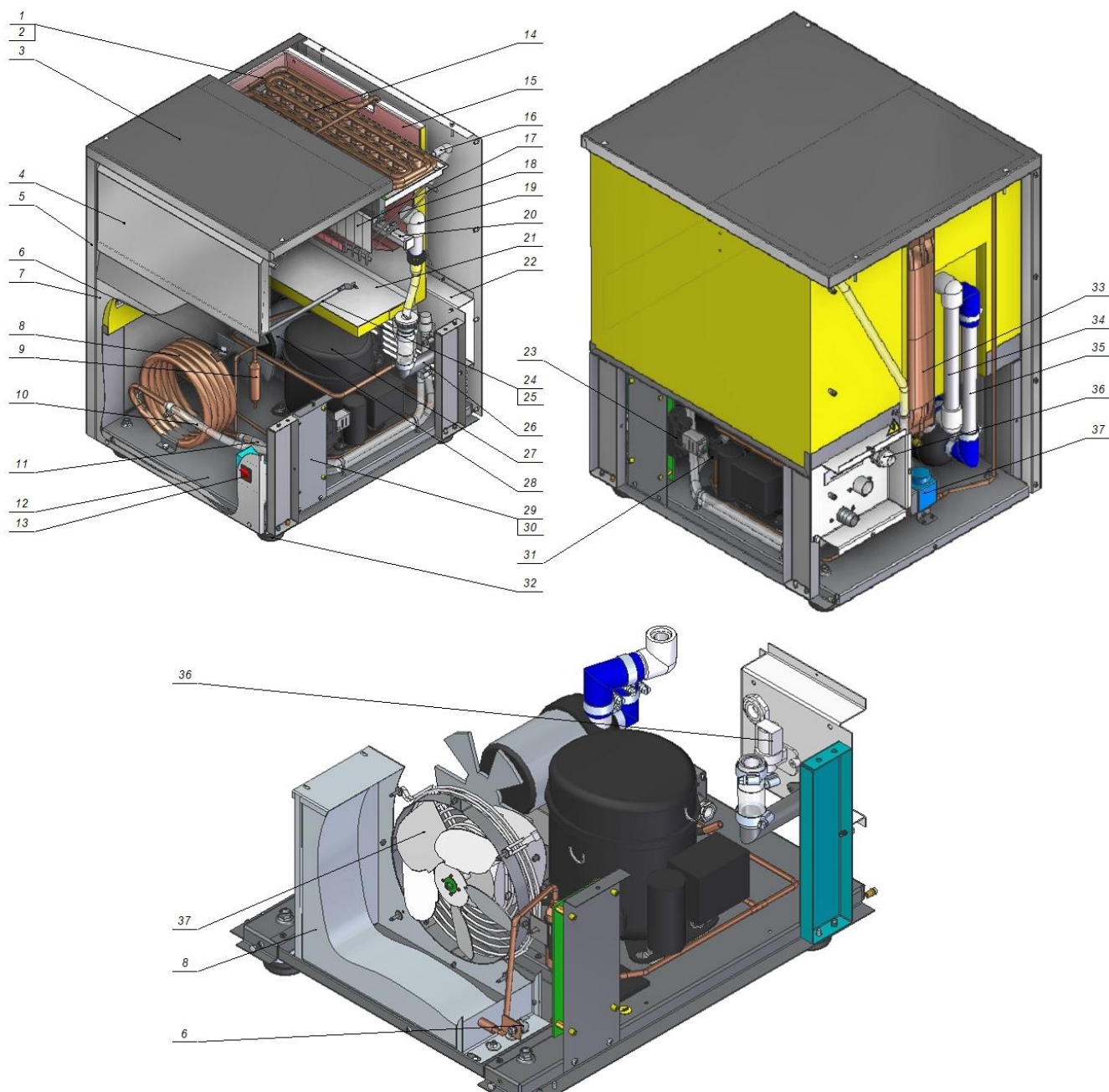
Рис. 1 Устройство льдогенераторов
