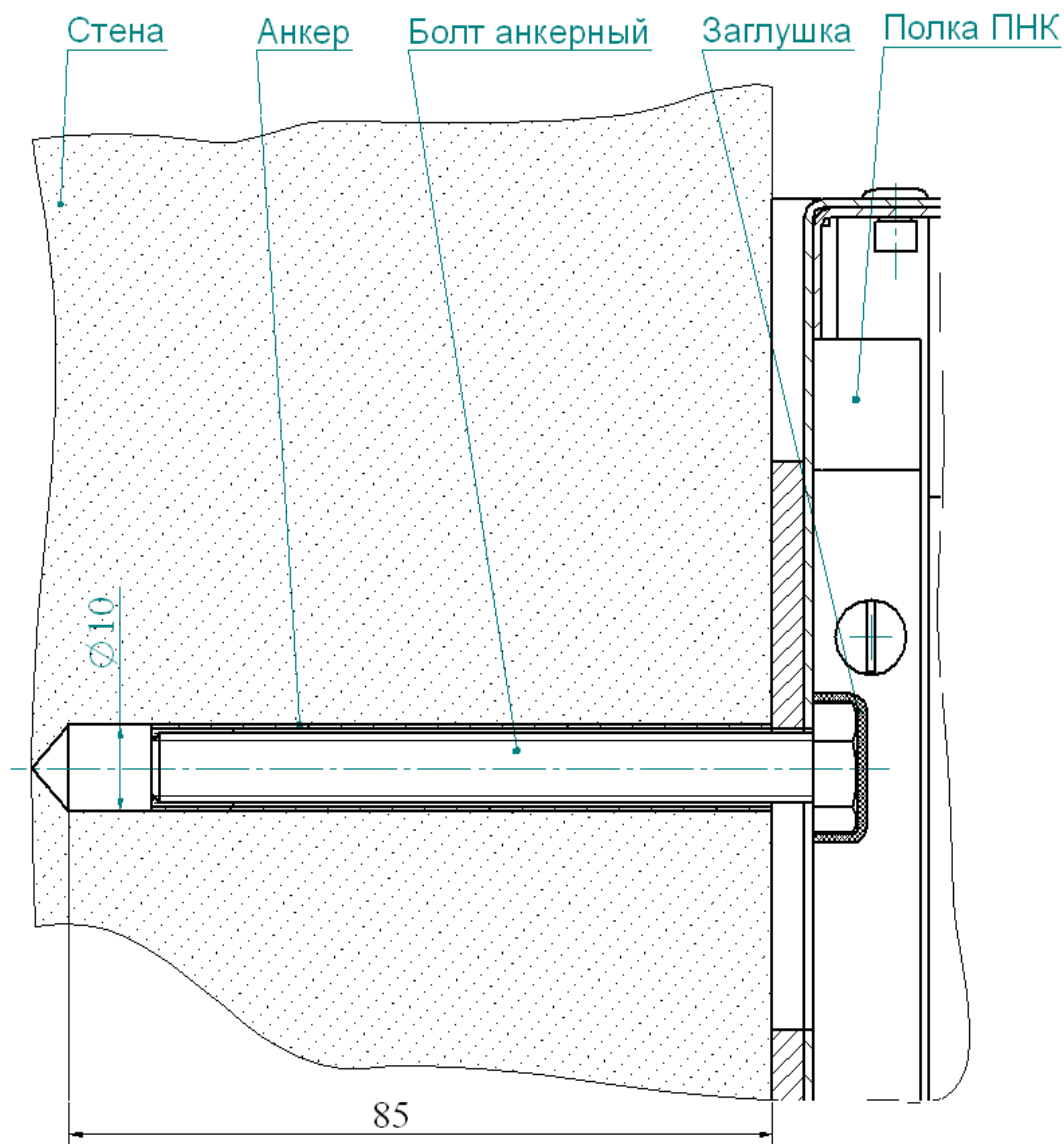
Рисунок 1. Пример крепления полки ПНК.
