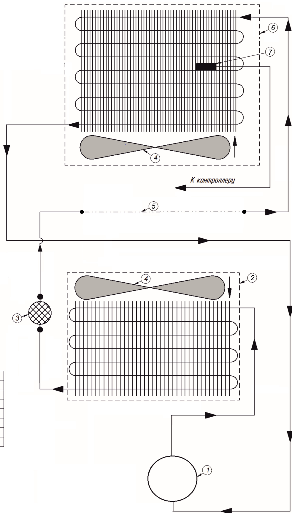
Рис. 9 Принципиальная схема системы охлаждения ШХн-0,5; ШХн-0,5-01;
