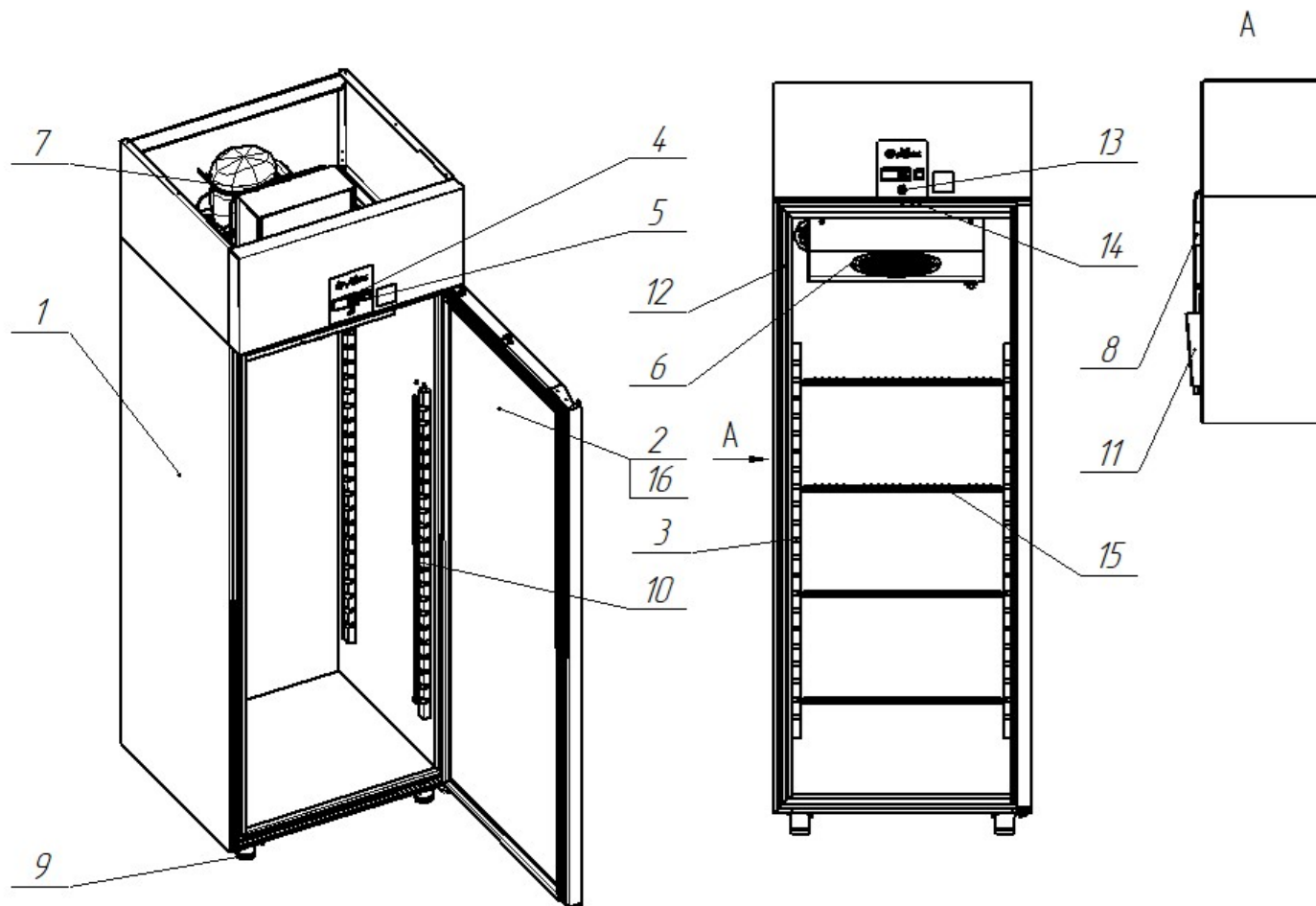
Рис. 3 Устройство шкафа ШХн-0,5; ШХн-0,5-01; ШХн-0,7; ШХн-0,7-01
