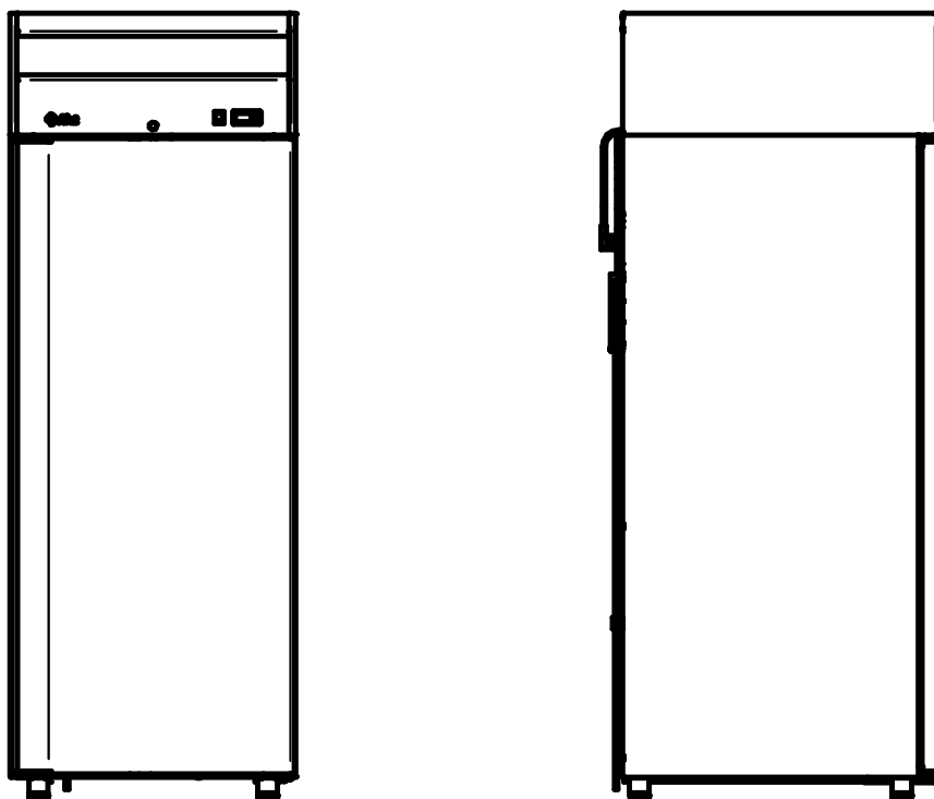
Рис. 1. Общий вид ШХн-0,5; ШХн-0,5-01; ШХн-0,7; ШХн-0,7-01 с верхним расположением АКК
