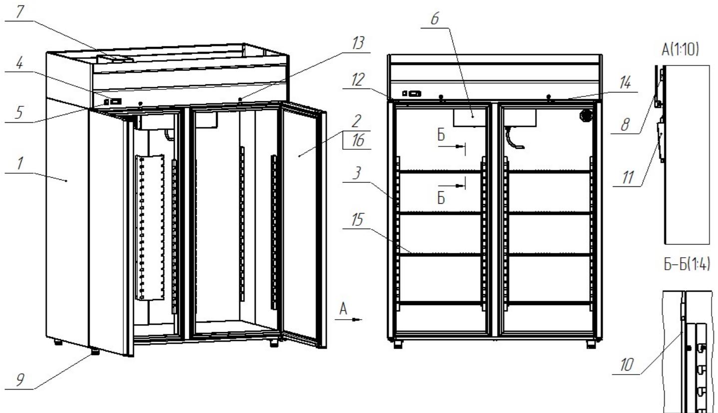
Рис. 4 Устройство шкафа ШХн-1,4; ШХн-1,4-01
