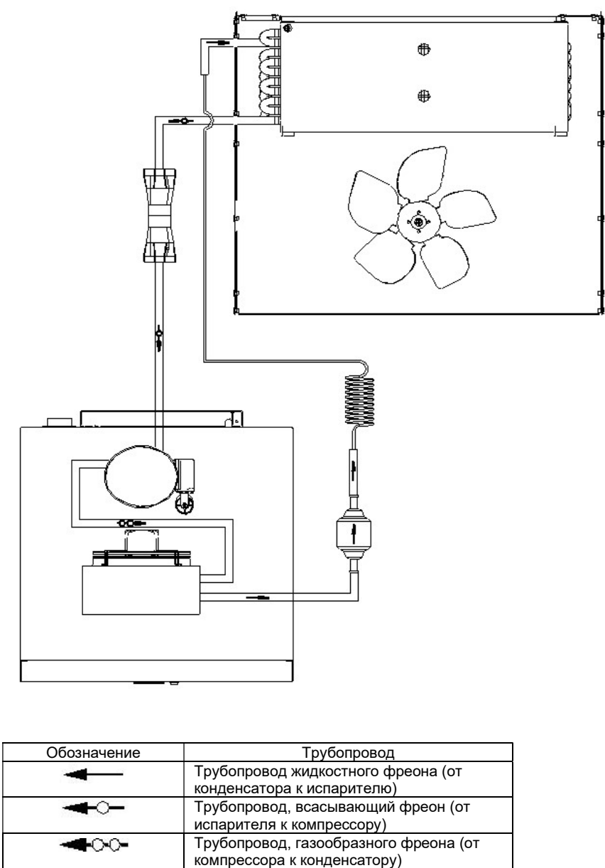
Рис. 7 Функциональная схема системы охлаждения ШХн-0,5; ШХн-0,5-01; ШХн-0,7; ШХн-0,7-01
