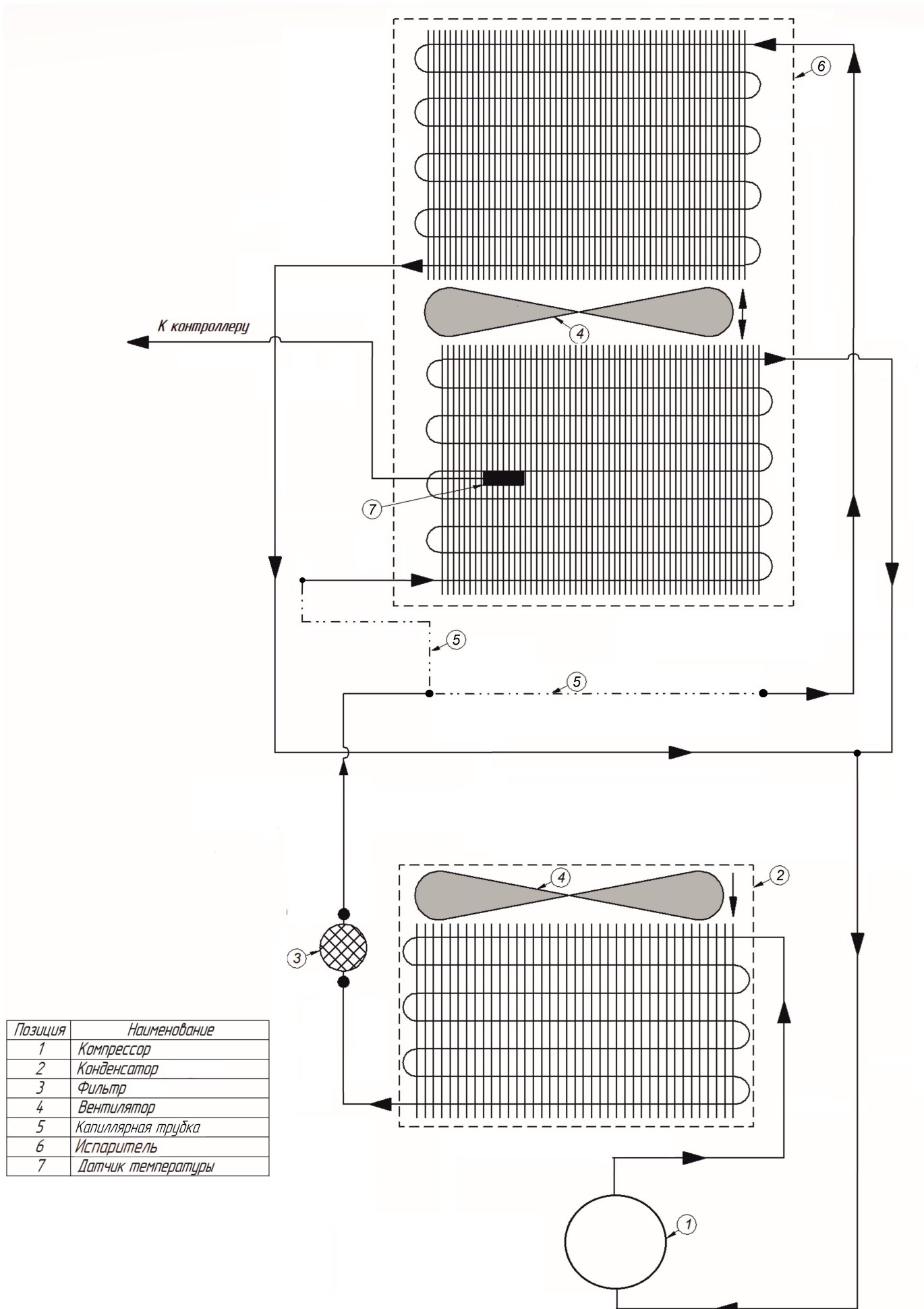
Рис. 10 Принципиальная схема системы охлаждения ШХн-1,4; ШХн-1,4-01;
