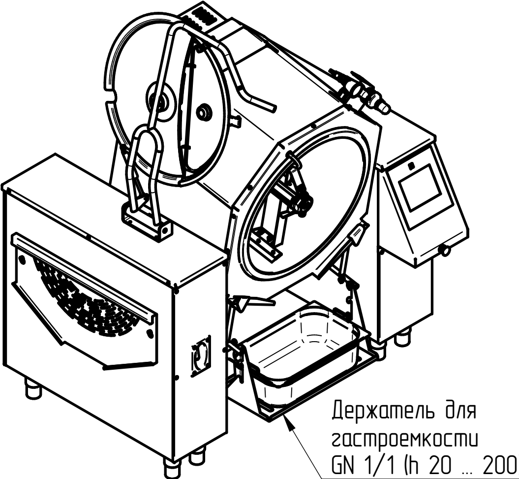
Котел в наклонном состоянии – 100°
