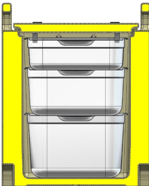
Рисунок 3 – Расположение гастроемкостей
