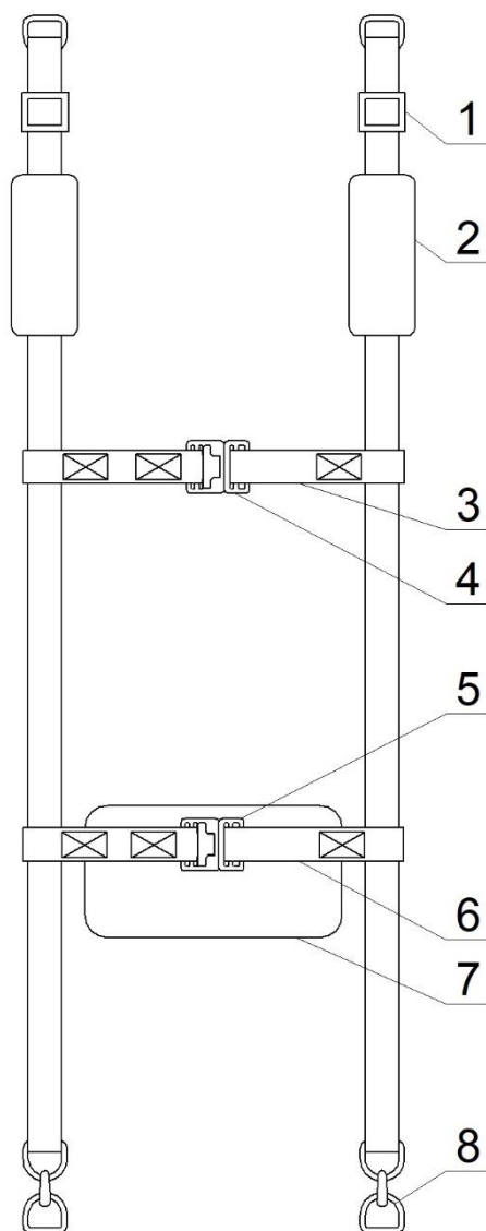
Рисунок 4 – Схема ременной системы
