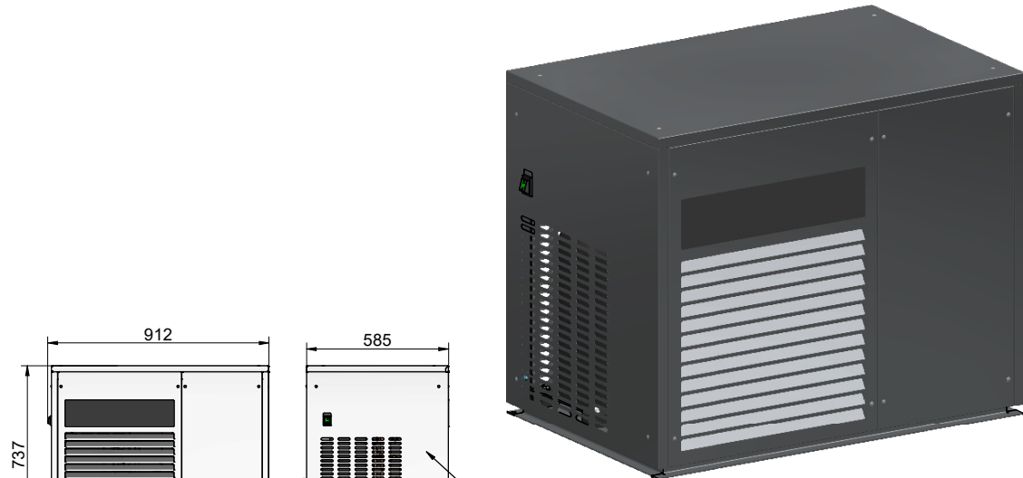
Льдогенератор ЛГ-400Ч-01/-02
