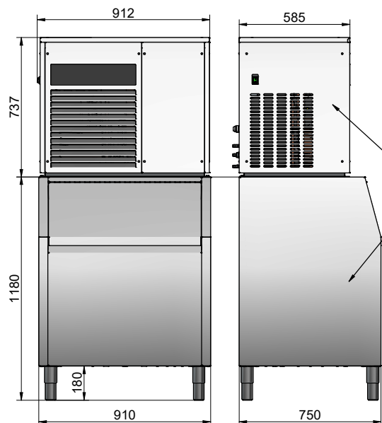
Льдогенератор ЛГ-400Ч-01/-02
