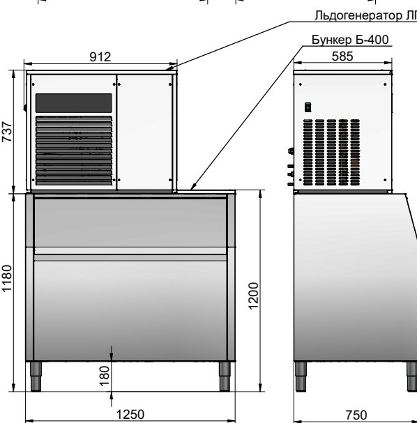
Льдогенератор ЛГ-400Ч-01/-02
