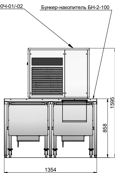
Бункер Б-400
