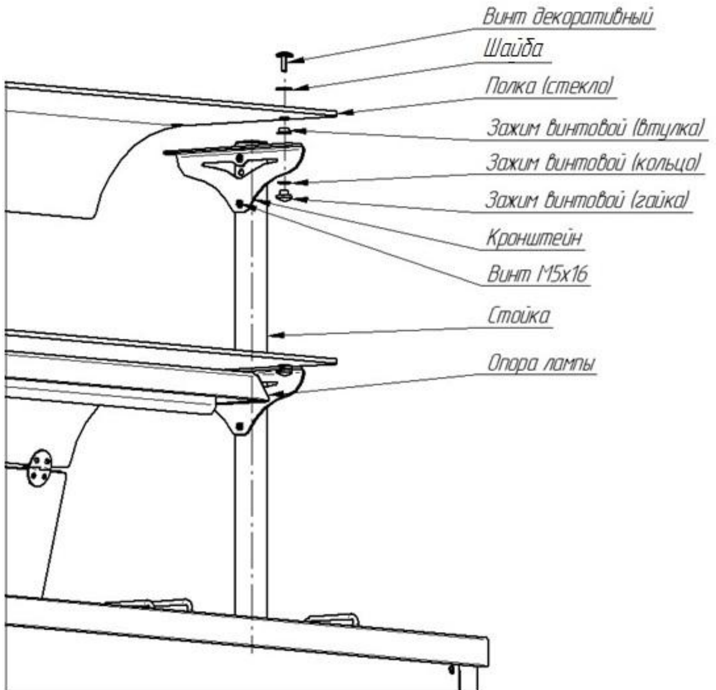
Рис.2 Сборка полок.
