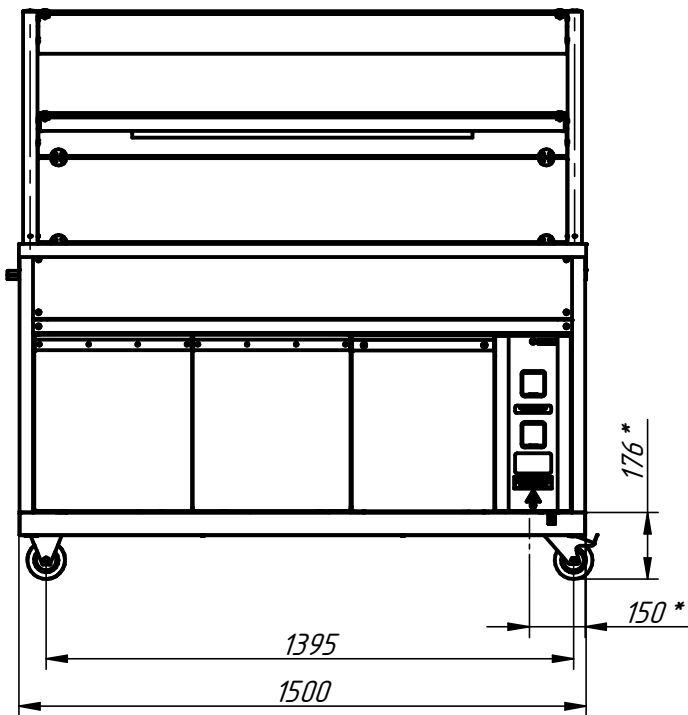
Вариант с поворотными колесами
