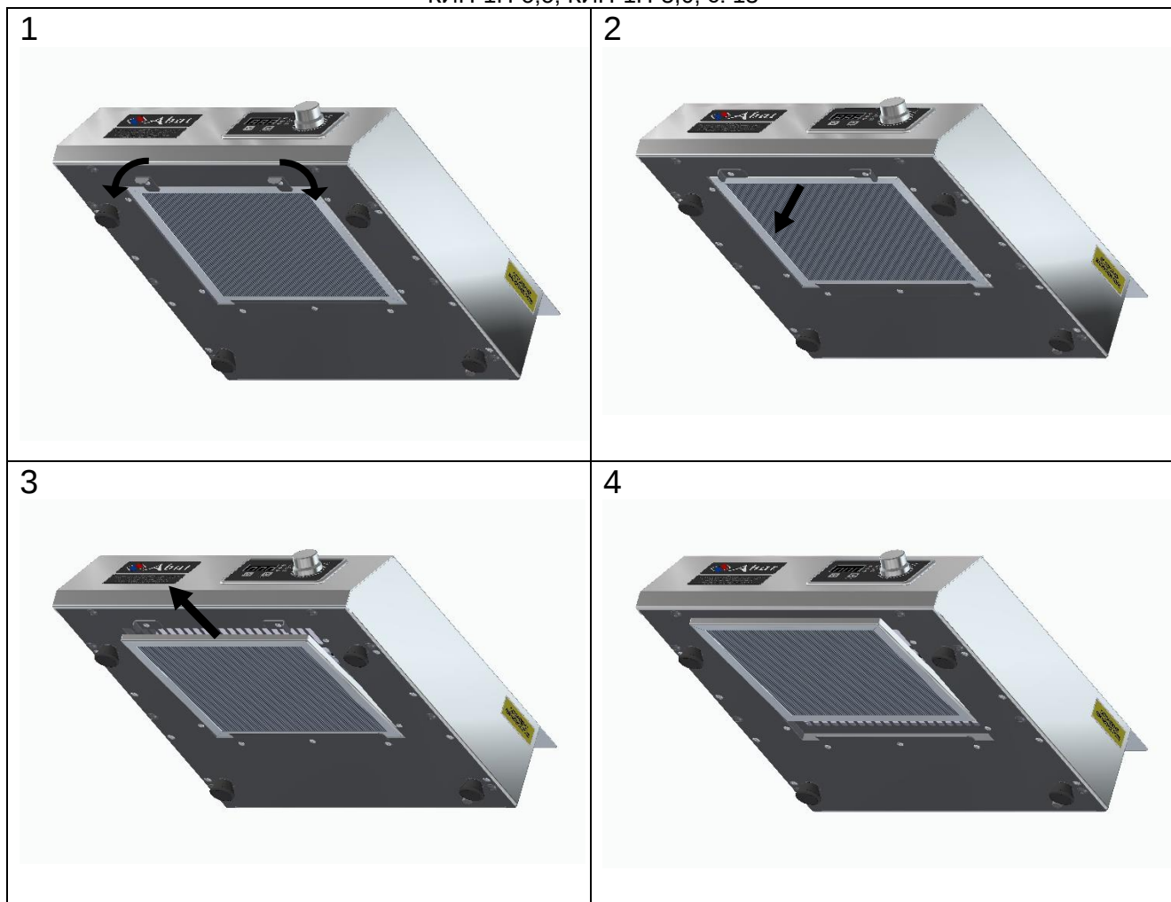
Рис. 4. Извлечение жирославливающего фильтра
