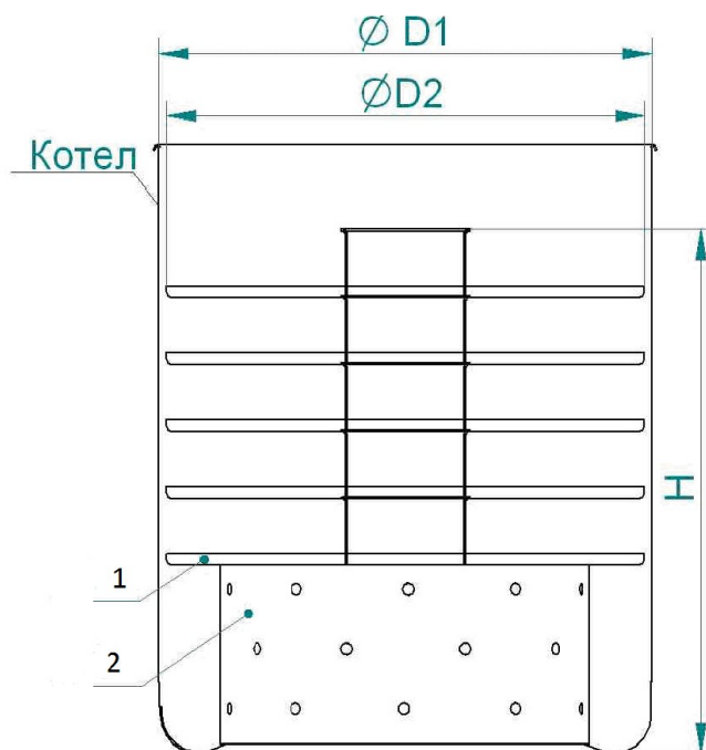
Рис. 1 1 - Секция, 2 – Основание
